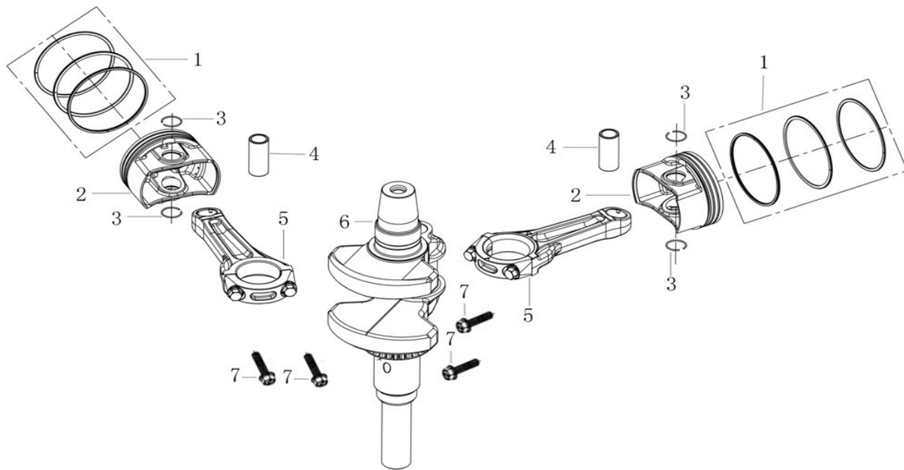
曲轴_活塞 ( CRANKSHAFT_PISTON )
