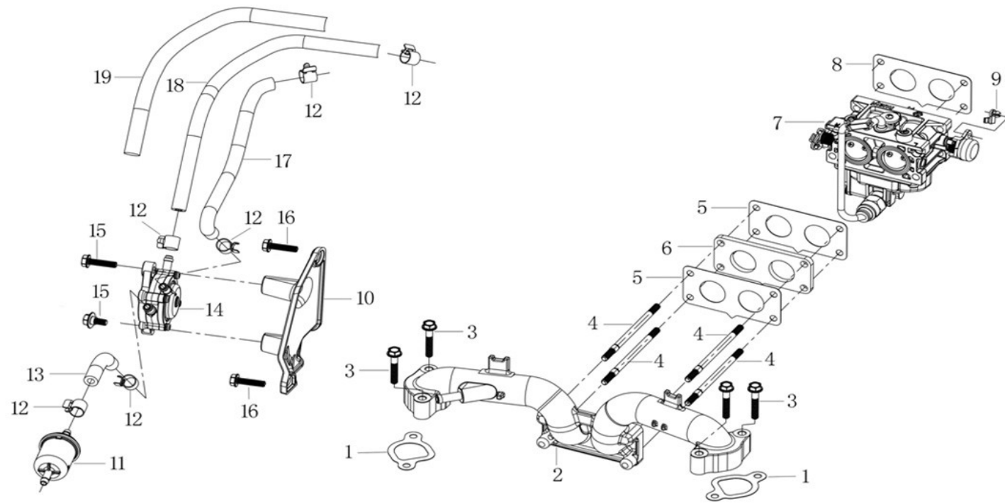
化油器 ( CARBURETOR )
