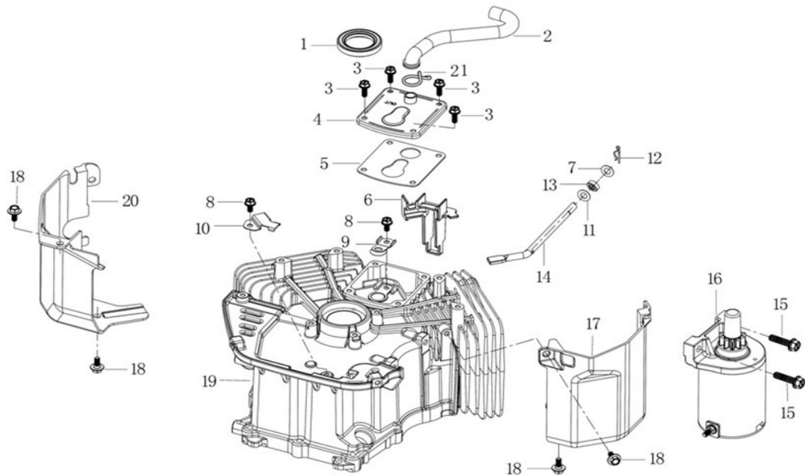
曲轴箱体 ( CRANKCASE )
