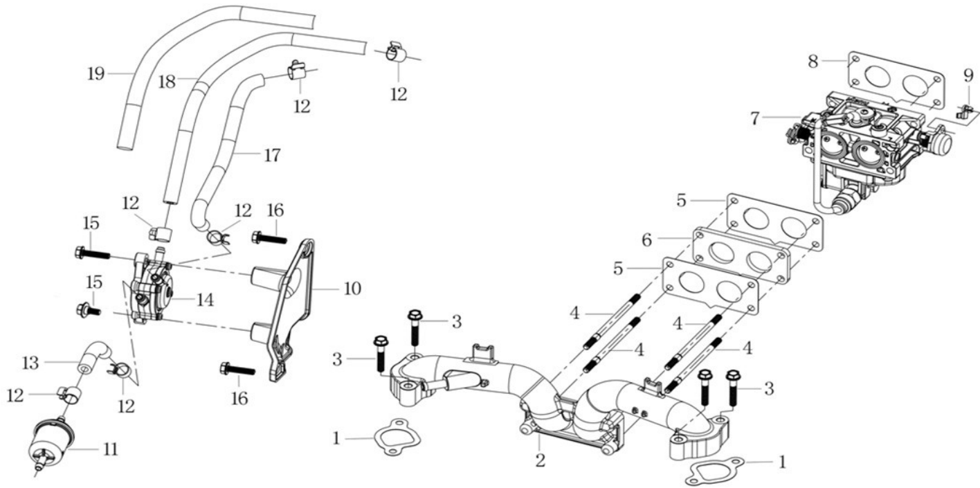
化油器 ( CARBURETOR )
